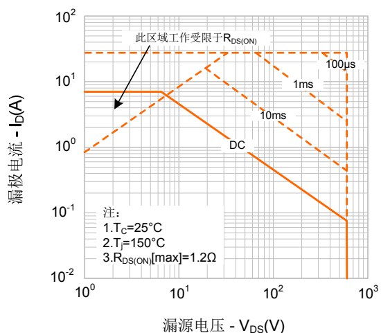
图9-1. 最大安全工作区域(SR 7N65F)
