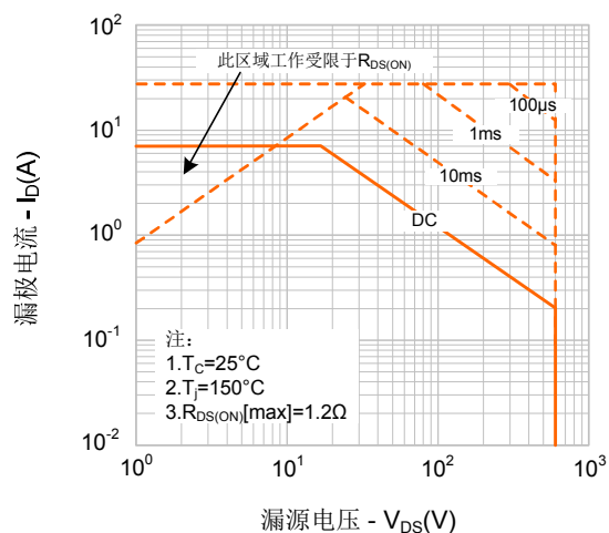
图9-2. 最大安全工作区域(SR 7N65S)
