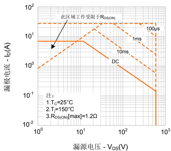
图9-3. 最大安全工作区域(SR 7N65D)
